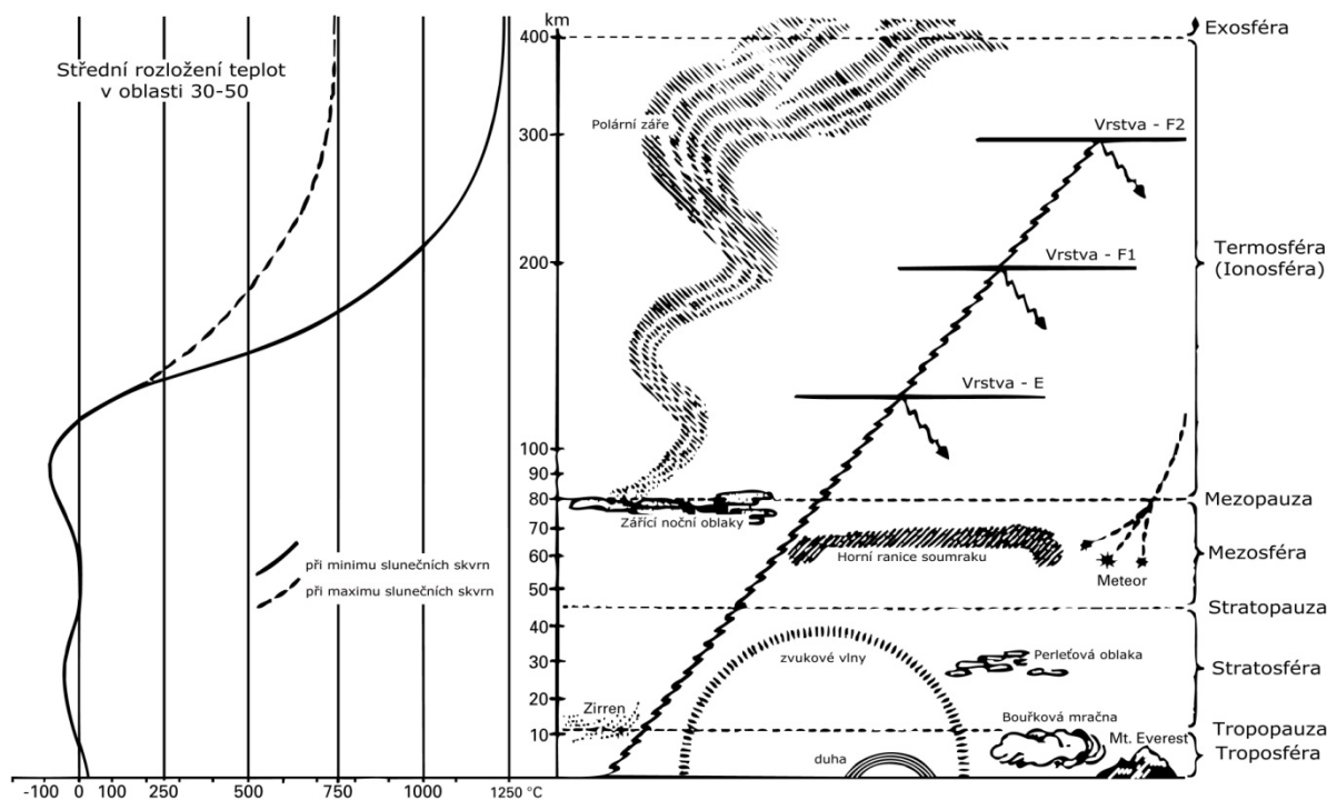
Struktura a střední teplotní rozložení pozemské atmosféry
